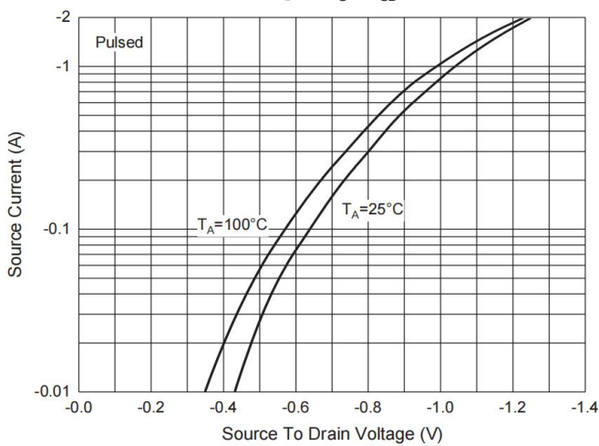
Fig. 3 - I_S - V_{SD}
